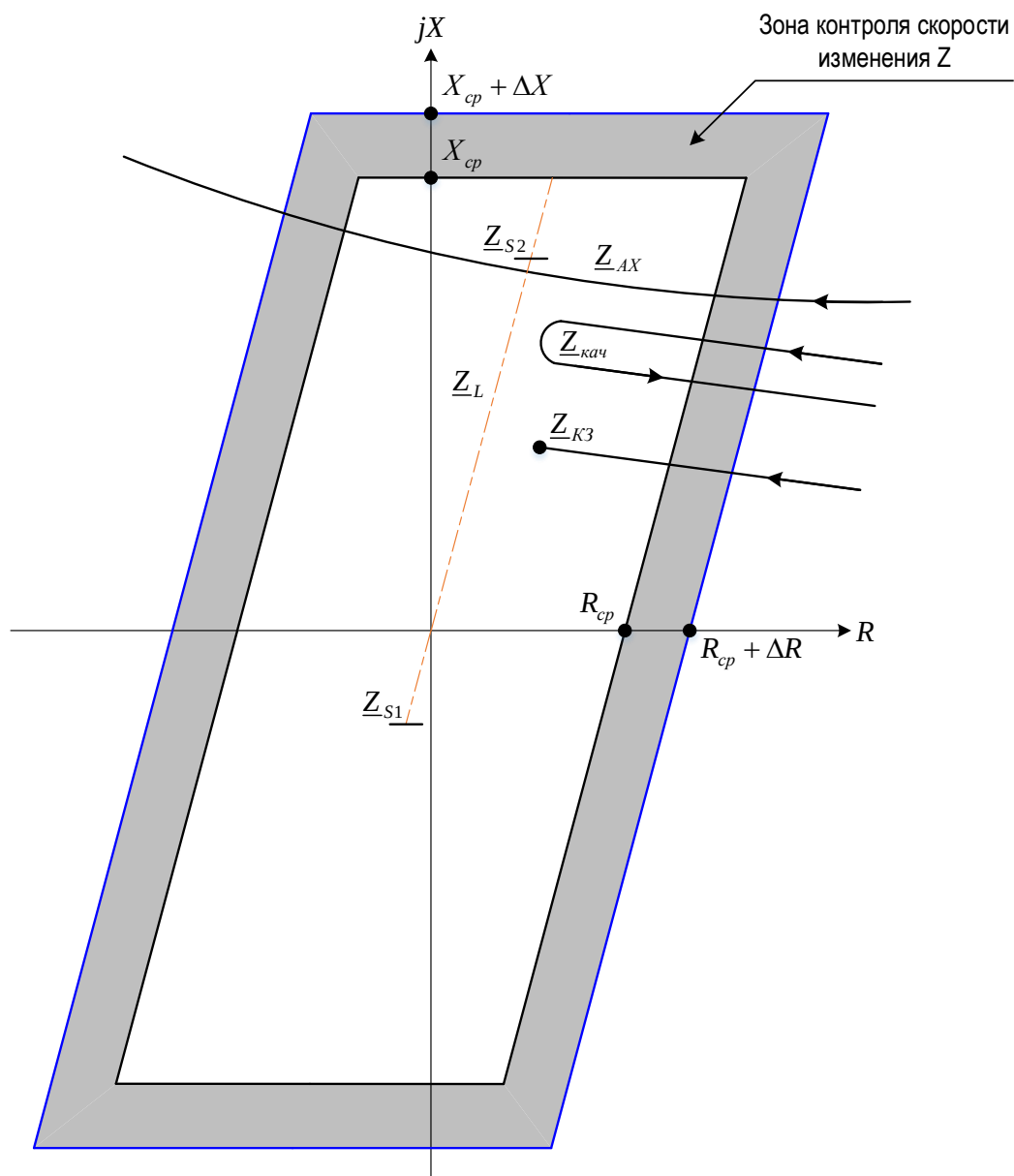
Рисунок 1.18 – Характеристики реле сопротивления, используемые для блокировки при качаниях по скорости изменения сопротивления
