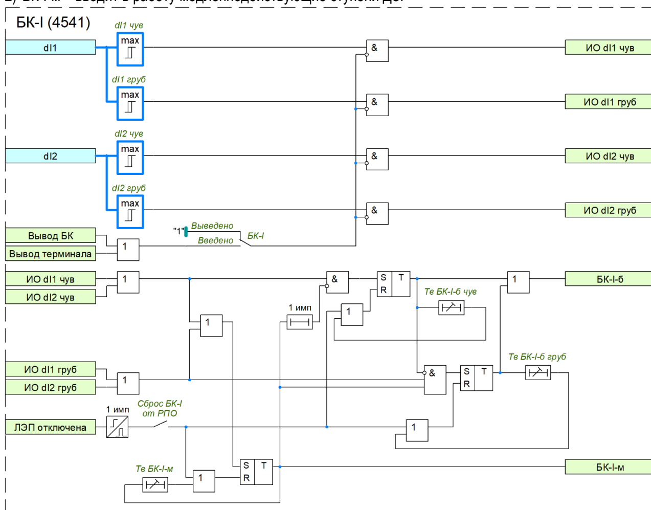
Рисунок 1.15 – Функциональная схема пуска БК-I
