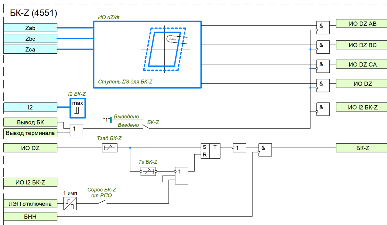
Рисунок 1.17 – Функциональная схема БК-Z
