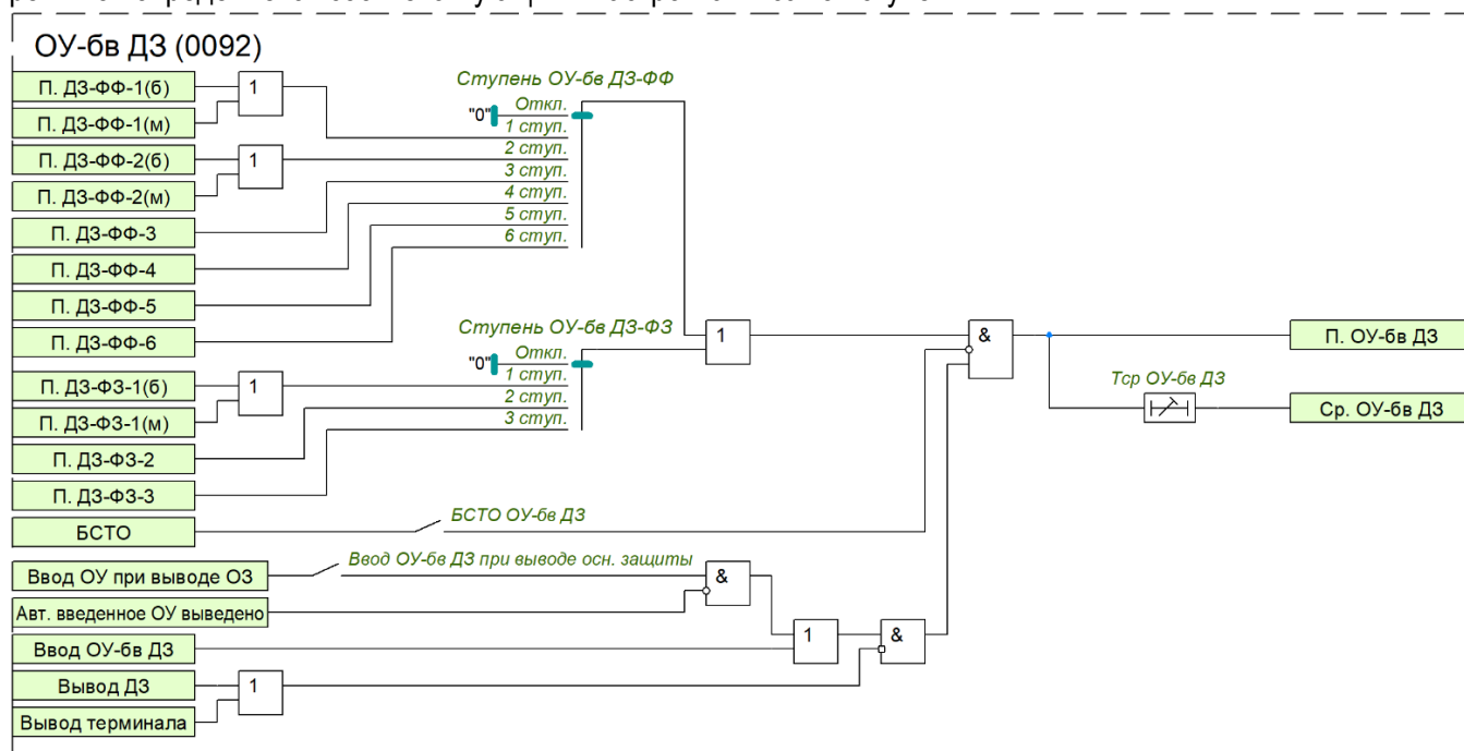
Рисунок 1.14 – Функциональная схема ОУ-бв ДЗ
